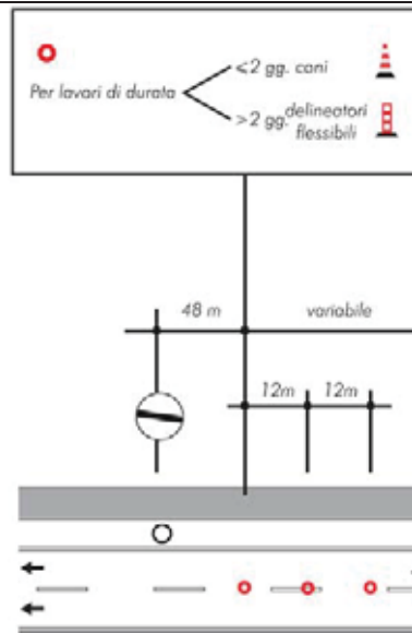
fig. 9 Segnaletica di posizione – delimitazione longitudinale e segnale di fine prescrizioni
